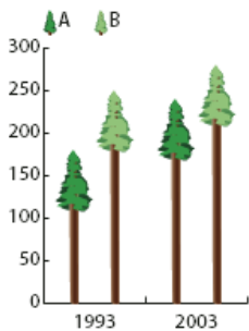
Symbole à proportion partielle
