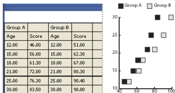
Données d'un graphe à nuages de points
