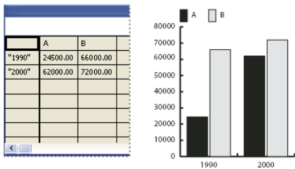
Données d'un graphe à barres verticales
