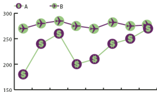
Graphe linéaire avec symboles de point
