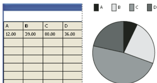
Données d'un graphe sectoriel
