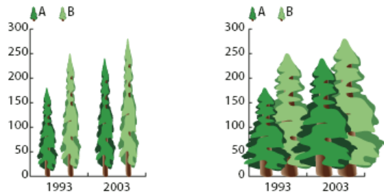
Comparaison entre un symbole de graphe à proportion verticale et un symbole à proportion uniforme
